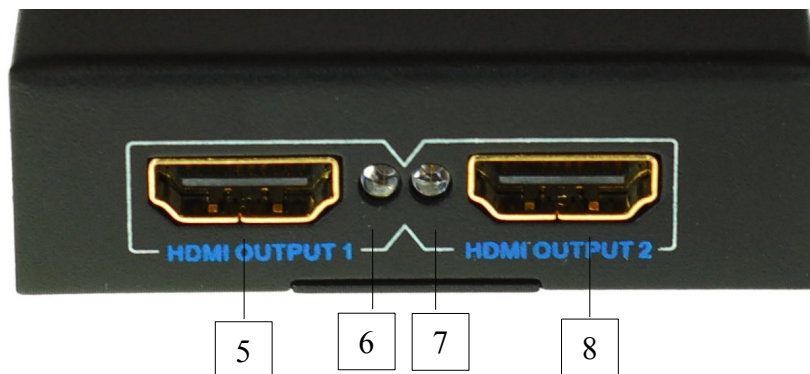
Bild 2: Rückansicht
